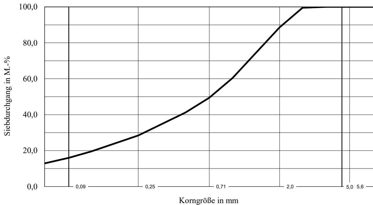
Abbildung 1: Korngrößenverteilung
