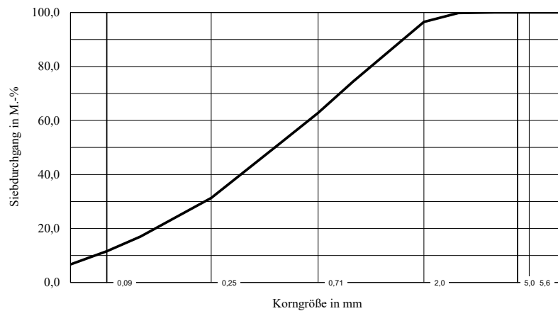
Abbildung 1: Korngrößenverteilung
